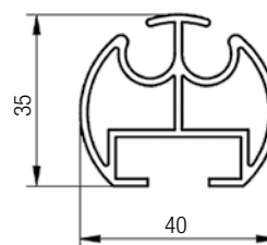
Sezione profilo box 250
