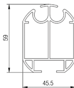
Sezione profilo box 500
