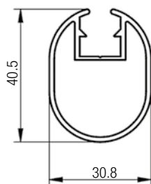
Sezione profilo trasversi
