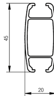
Sezione profilo perimetro
