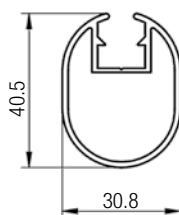
Sezione profilo
