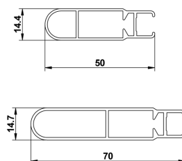
Sezione profili
