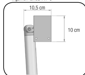
Ingombri tenda TTP 3
